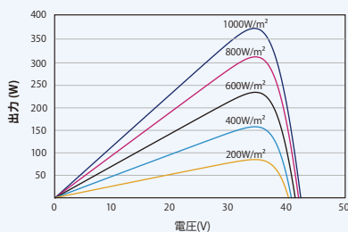
PVモジュール(375W)のPV曲線
